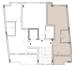
POLOŽAJ STANA NA OSNOVI POTKROVLJA
